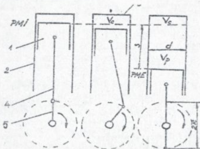
Fig.3.1. Parametrii principali ai unui motor.
